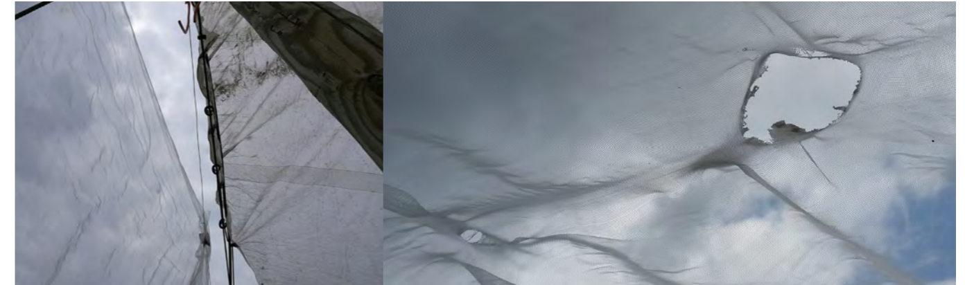
Abb. 27 und 28: Lücken zwischen Folienüberdachung und Netz müssen geschlossen werden; Löcher können als Eintrittspforten für die Fliege dienen Fotos: Augel/LTZ
