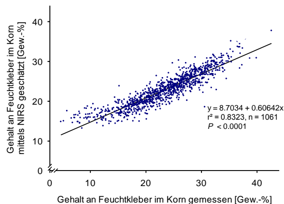
Abbildung 57: Schätzergebnis des NIRS-Verfahrens hinsichtlich des Gehaltes an Feuchtkleber im Korn im Vergleich zum Standardverfahren der Auswaschung des Feuchtklebers (geschätzt mit interner Standardkalibration des Infratec™ 1241-NIRS-Gerätes zur Ganzkornanalyse)
