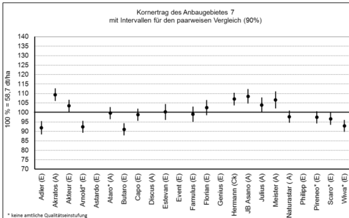
Abbildung 26: Schätzwerte für Kornertrag und 90 %-Vertrauensintervalle für paarweise Vergleiche der Kornerträge im ABG 7 (einschließlich Nachbargebiet 6) nach Hohenheim-Gülzower Serienauswertung (2010 bis 2012)
