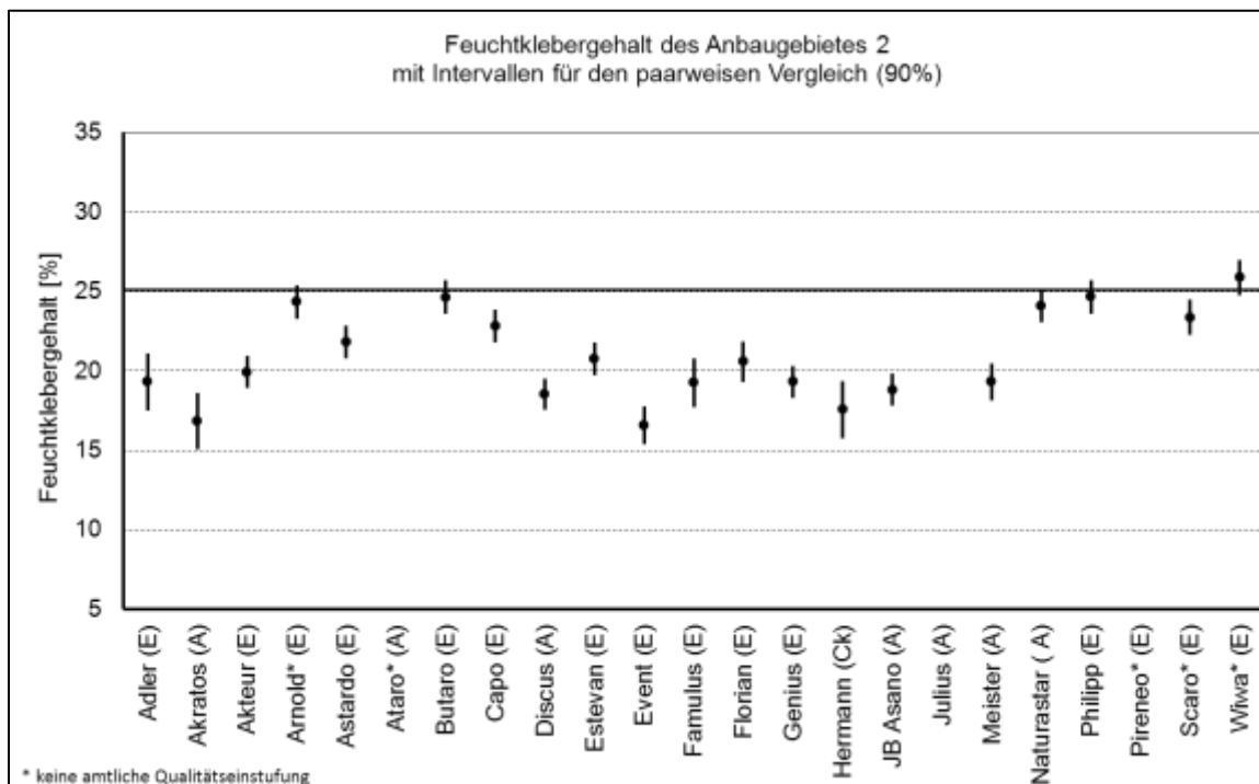
Abbildung 33: Schätzwerte für Feuchtklebergehalte und 90 %-Vertrauensintervalle für paarweise Vergleiche der Feuchtklebergehalte im ABG 2 (einschließlich Nachbargebiet 1) nach Hohenheim-Güzlöwer Serienauswertung (2010 bis 2012)
