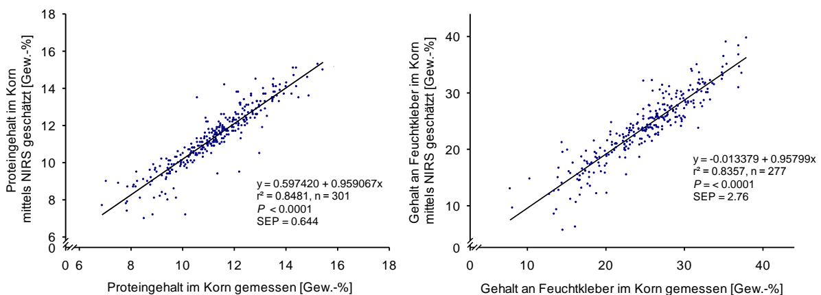
Abbildung 62: Schätzung des Kornproteingehaltes (links) und des Gehaltes an Feuchtkleber (rechts) im Winterweizenerntegut des Jahres 2012 anhand der neu erstellten Kalibrationsfunktionen
