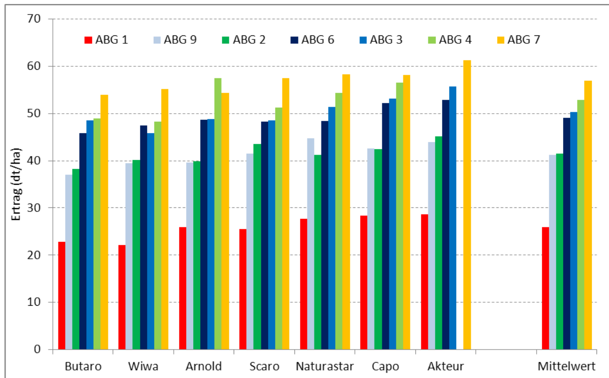
Abbildung 29: Kornerträge der Winterweizensorten des orthogonalen Sortiments in 7 Anbaugebieten (ABG) (2010 bis 2012)
