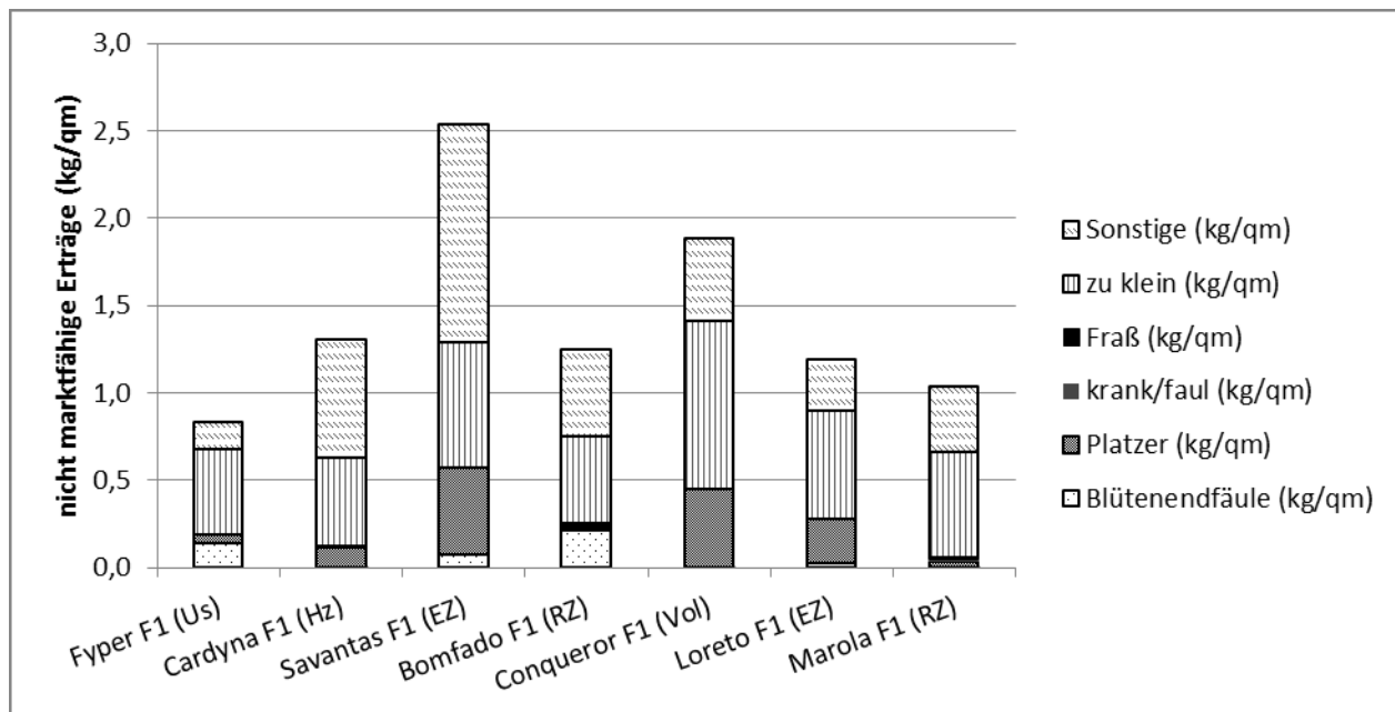
Abb. 2: Nicht marktfähiger Ertrag von Eiertomatensorten im ökologischen Anbau im kalten Folienhaus, aufgeschlüsselt nach Kategorien und sonstigen Qualitätsmängeln in kg/m 2 (Mittelwerte aus drei Wiederholungen).
