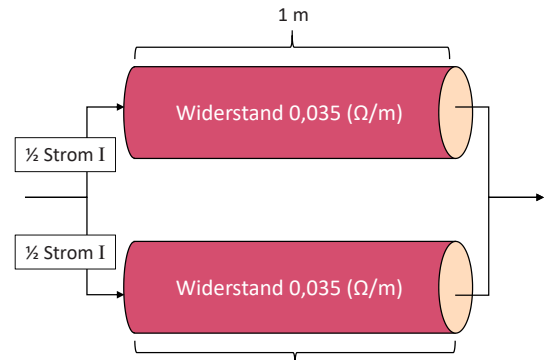
Gesamtwiderstand = \frac{1}{2} * 2 \text{ m} \times 0,035 \Omega/m = 0,035 \Omega Abb. 14: Durch Verdopplung der Leiterfläche (zwei Drähte statt einem) halbiert sich der Gesamtwiderstand der Anlage.
