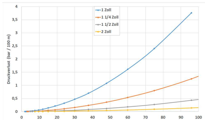
Abb. 6: Abhängigkeit des Druckverlusts (bar) je 100 m von Leitungsquerschnitt und Wassernachlauf (Liter / Minute) bei einem PE-Schlauch.
